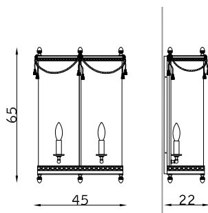
31124 2 x E14 30W
