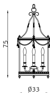
31121 3 x E14 30W
