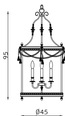
31120 3 x E14 30W
